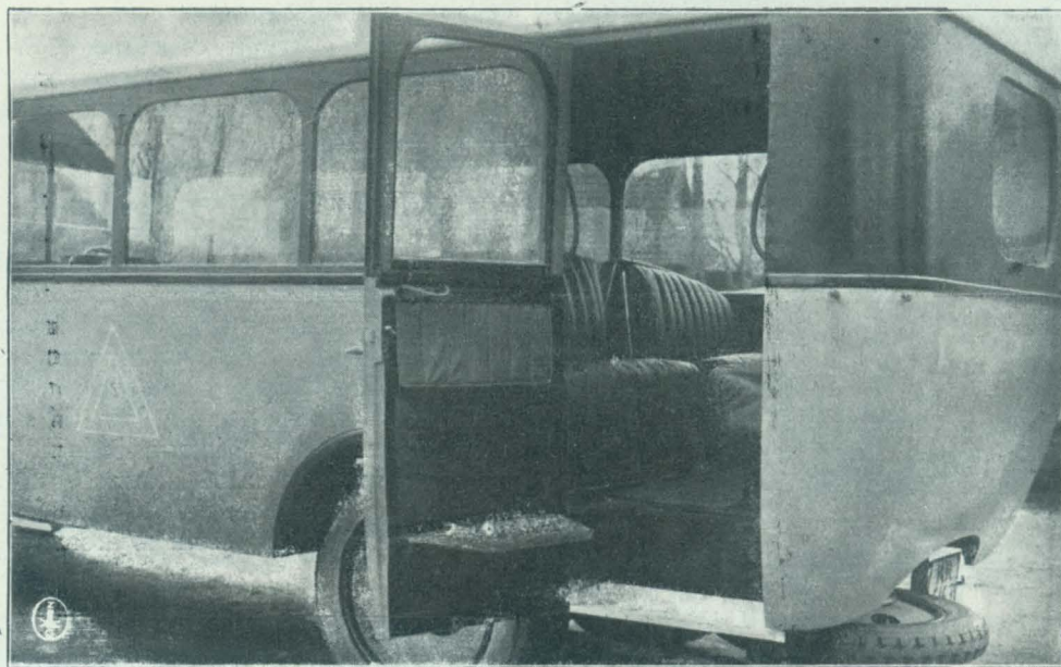
Detale pięknej karoserji wykonanej przez Zakopiańską Spółkę Samochodową.
