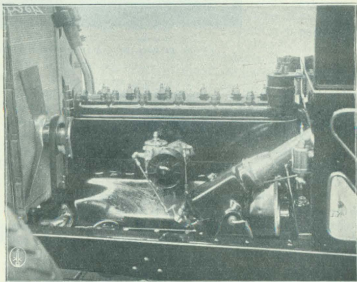
Z Salonu Brukselskiego. Silnik 29 KM. MERCEDES.
