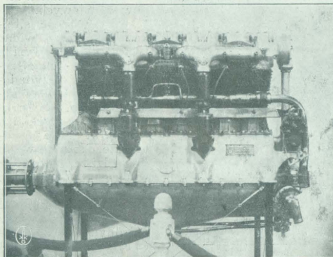
Salon Lotniczy w Paryżu. Najciekawsze silniki: 1) Salmson 630 KM. 2) Jupiter 500 KM. 3) Lorraine-Dietrich 450 KM. (18 cylindrów). 4) Lorraine 500 KM. (12 cylindrów). 5) Farman 700 KM. 6) Isotta Fraschini 180 KM. 7) Renault 480 KM.
