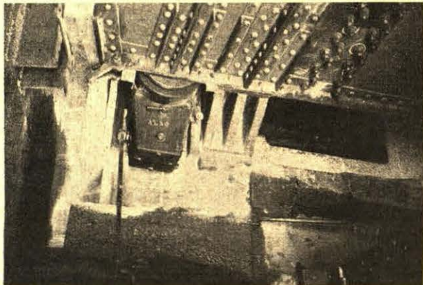
Rys. 10. Wymiana łożysk.
