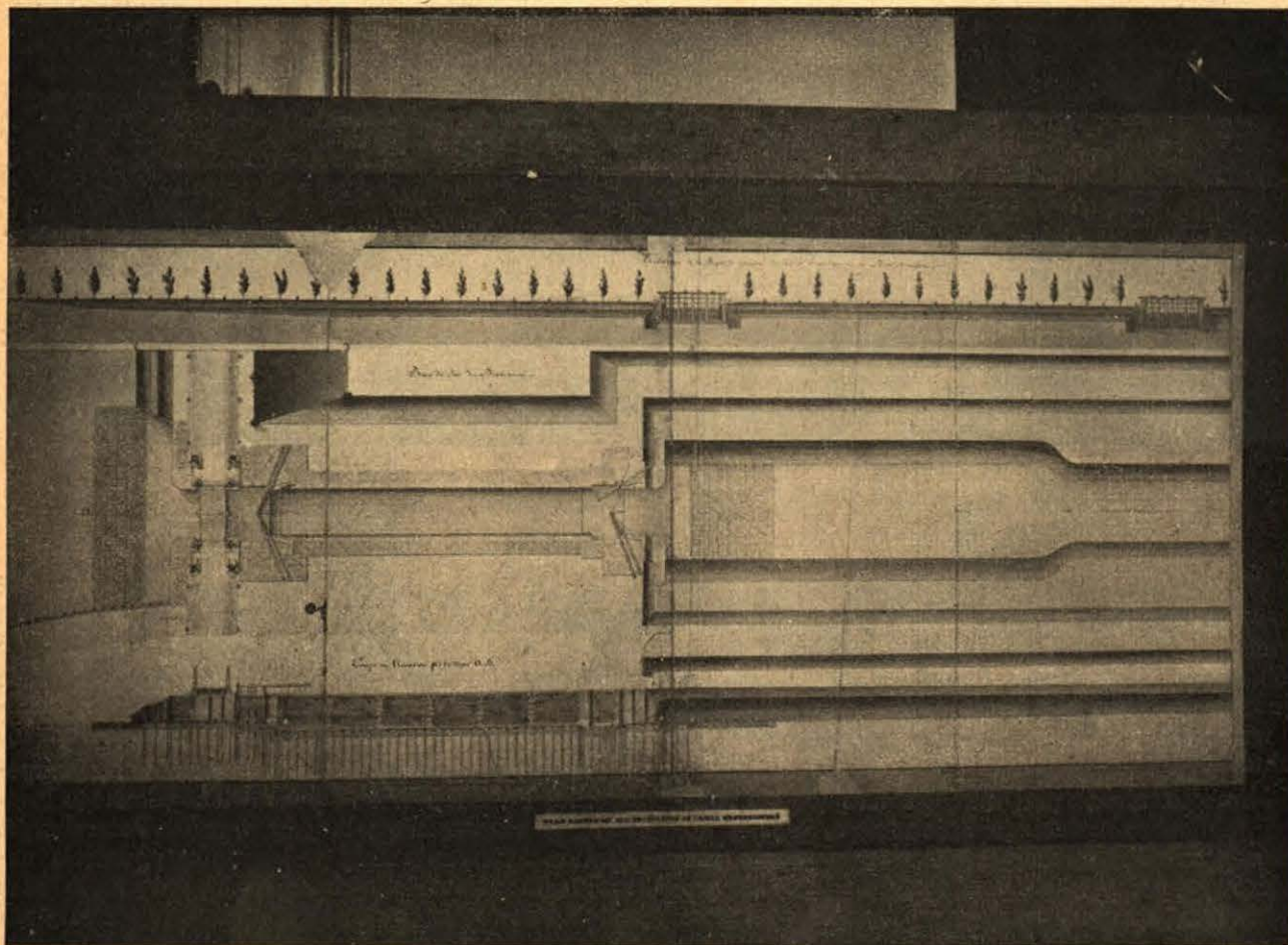
Plan ancien de 1827 des écluses du canal Augustowski.
