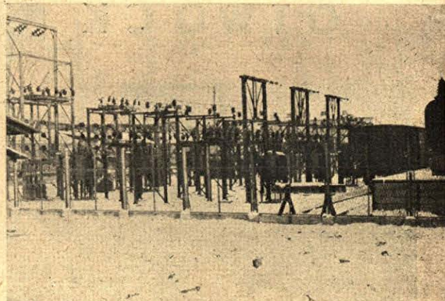
Rys. 3. Podstacja.
