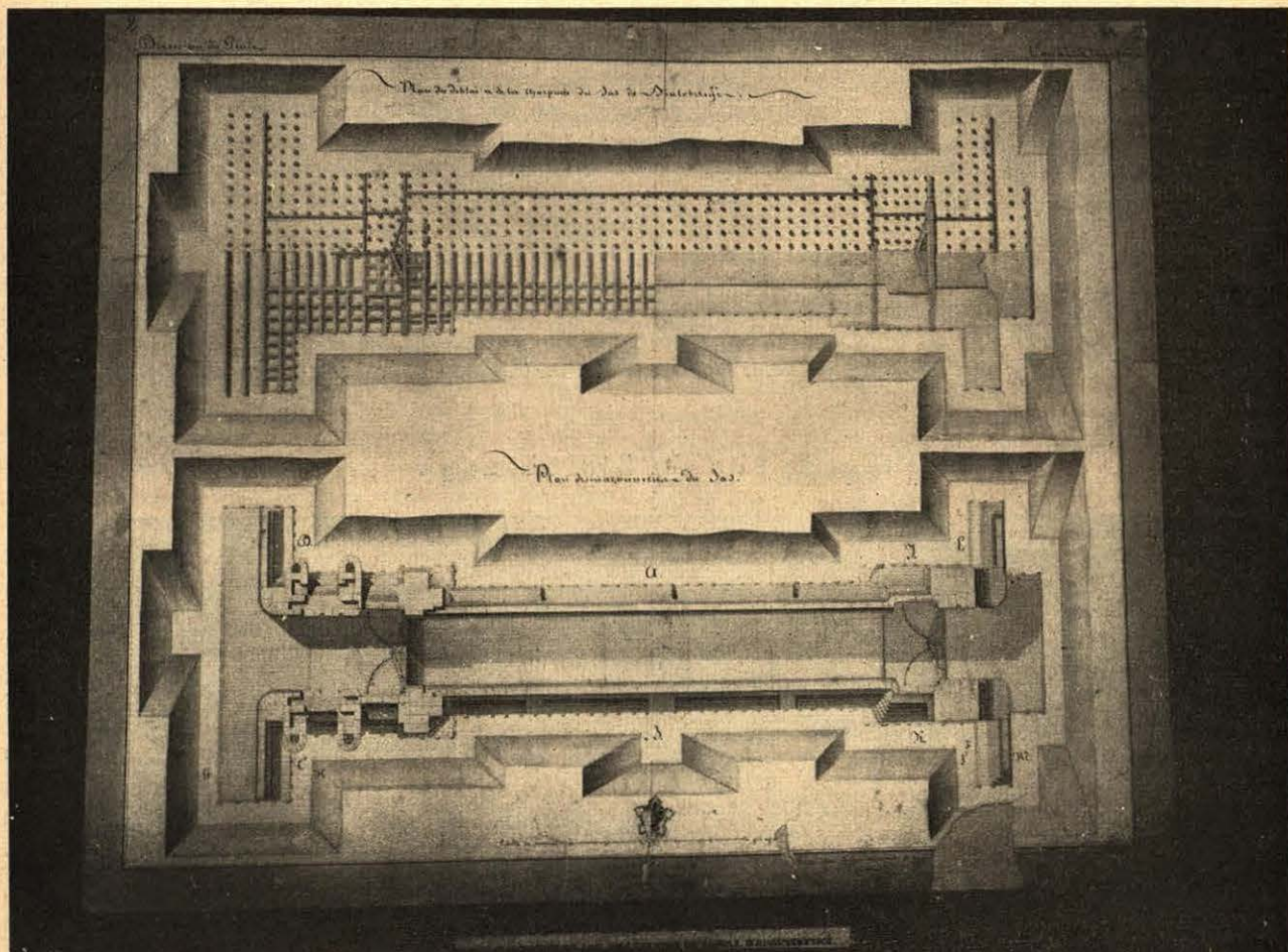
Rys. 4. Plan ancien de 1827 des écluses du canal d'Augustowski.
