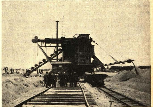
Rys. 2. Czerparka (t. zw. bagier) w czasie pracy.
