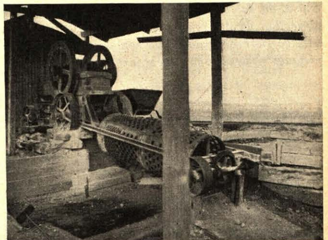
Rys. 3. Łamacz kamienia.
