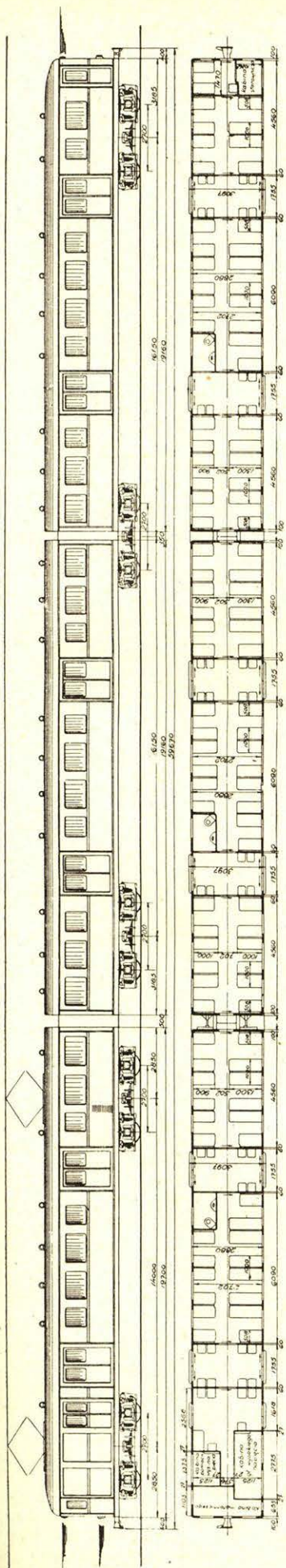
Rys. 2. Zespół trójczłonowy wagonów elektrycznych, budowany przez wytwórnię Lipop, Rau i Loewenstein i H. Cegielski oraz Zieleniewski i Fitzner-Gamper.
