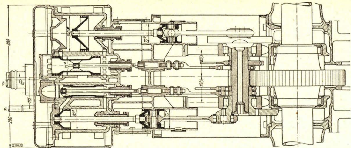
Rys. 15. Szybkobieźna maszyna parowa suwakowa (1500 obr./min. do wysokoprężnych wagonów parowych typu Doble'a).
