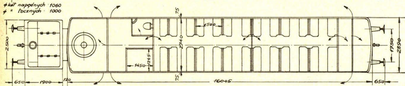
Rys. 12. Wagon parowy systemu Clayton'a, zbudowany przez wytw. H. Cegielski.
