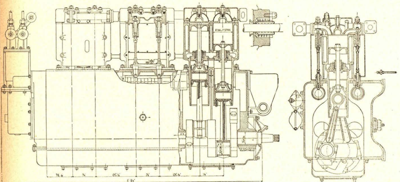
Rys. 7. Sześciocylindrowa maszyna parowa jednostr. dział. wagonu syst. Sentinel-Cammel'a.
