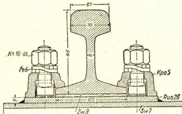
Rys. 9. Niemiecka nawierzchnia „K” na podkładach stalowych. Płytkę podkładową przypawana.
