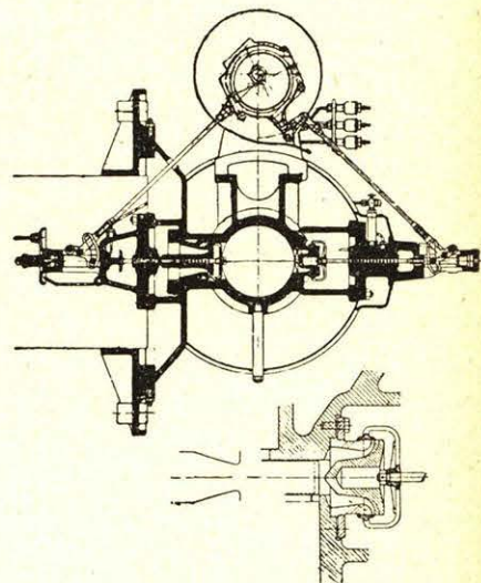
Rys. 18. Przekrój maszyny parowej syst. Gutmuth'a, z zaworami dyfuzorowemi.
