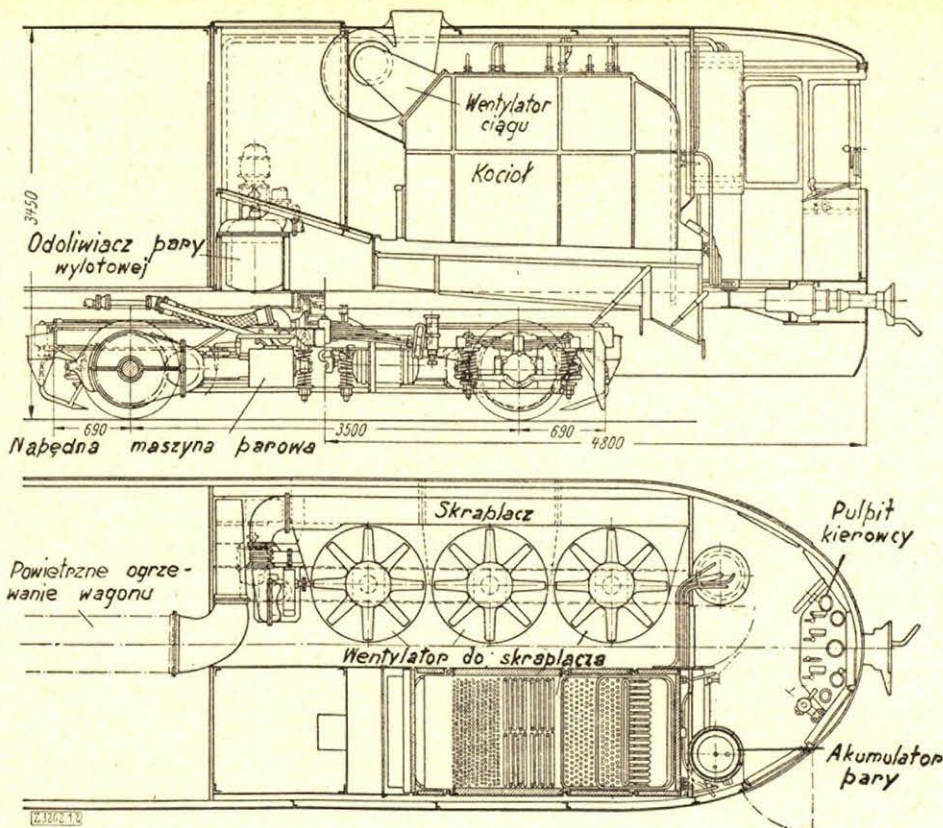
Rys. 19. Układ urządzeń napędowych w wagonie parowym w/g projektu Krupp'a.
