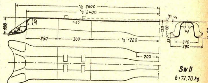
Rys. 7a. Podkład stalowy kolei oldenburskich według propozycji Vogla.
