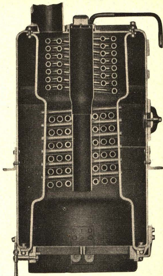
Rys. 3. Przekrój kotła syst. Clayton'a z górnym zasilaniem paleniska (w wagonie zakupionym w Anglii).
