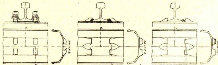
Rys. 16. Różne rodzaje umocowania szyny: a) nawierzchnia niem. „K” b) naw. klinowa c) naw. z klinami owalnymi.
