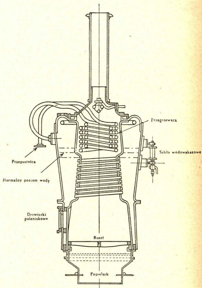
Rys. 4. Przekrój kotła syst. Clayton'a z boczным zasilaniem paleniska w wagonie, zbudowanym przez wytwórnię H. Cegielski.
