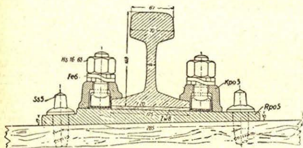
Rys. 8. Niemiecka nawierzchnia „K” na podkładach drewnianych. Uważę zwraca duża i ciężka podkładka.
