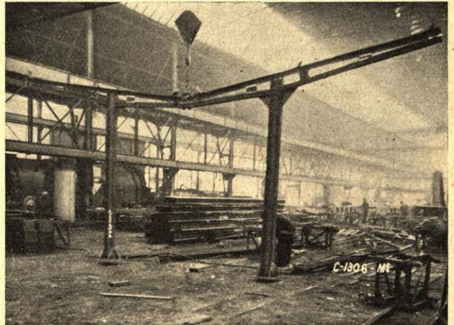
Rys. 7. Więzar dwusłupowy (złożony w warsztacie).
