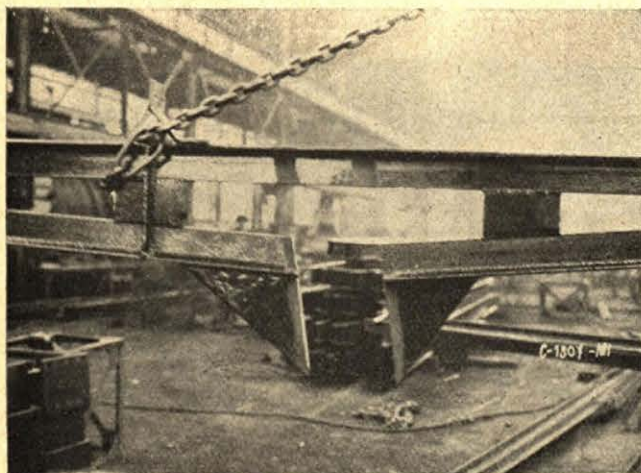
Rys. 8. Połączenie rozpory z słupem w więźarze dwusłupowym.
