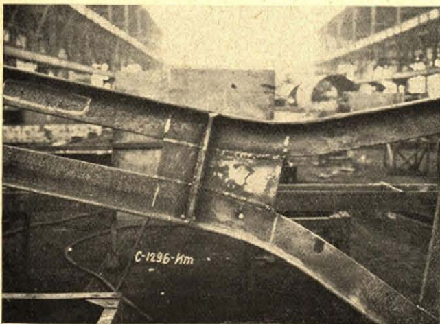
Rys. 10. Szczegół podstawy więźara jednosłupowego.
