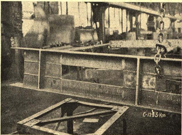
Rys. 5. Szczegół słupa więzara jednosłupowego.
