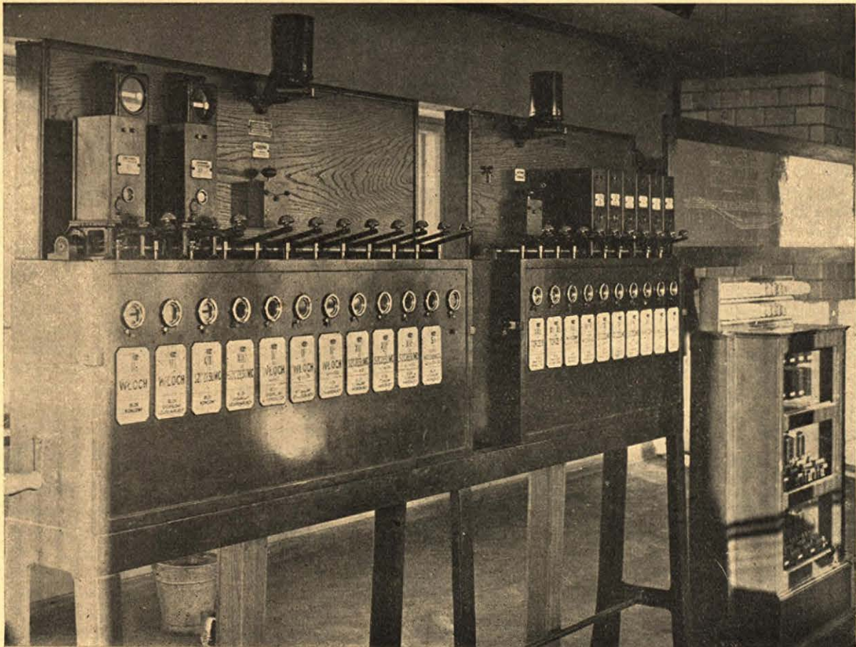
Rys. 2. Aparat blokowy.
