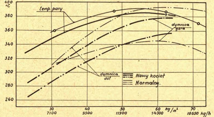
Temperatury pary przegrzanej i gazów i dymnicy. rozm. niemieckie
