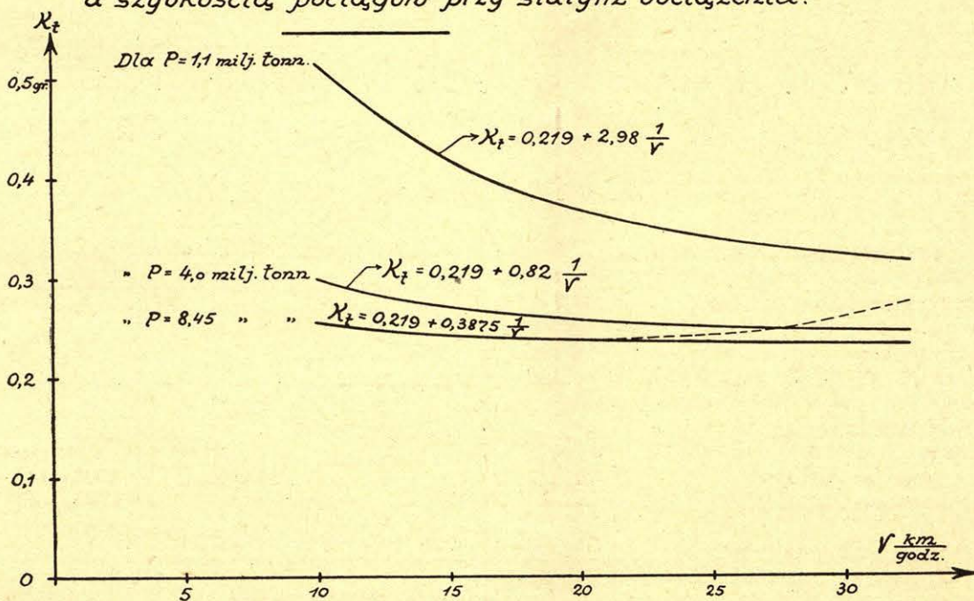
Rys. 5. Zależność wydatków st. trakcji na 1 tonno * km - br. a szybkością pociągów przy stałym obciążeniu.
