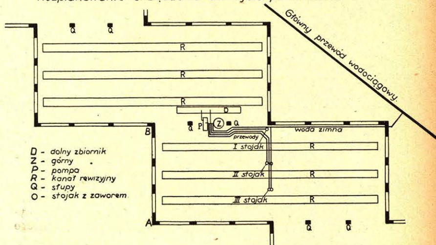
Rozplanowanie urządzenia do mycia parowozów.
