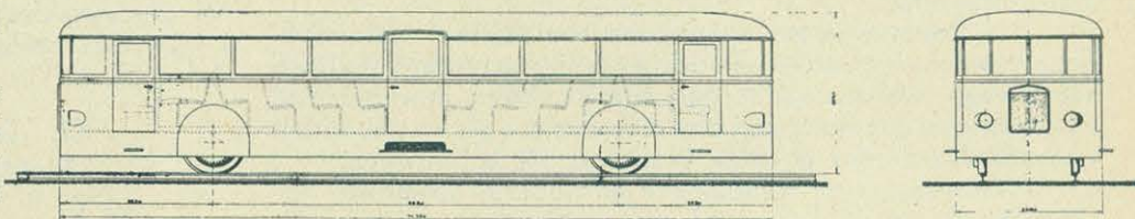
Autobus normalno-torowy dla 32 pas. Dwukierunkowy. Rozstaw osi 5,2 m. Cała długość ok. 10,24 m. Szybkość ok. 100 km/g.
