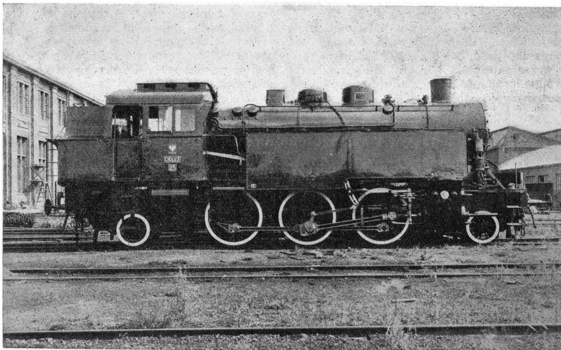
Rys. 1. Widok ogólny parowozu serji OK127
