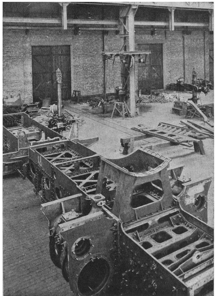
Rys 4. Widok zmontowanego podwozia parowozu serii OK127.
