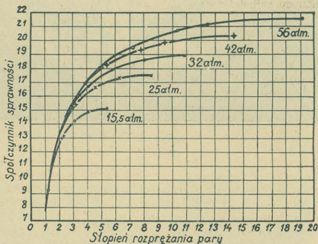
Zależność współczynnika sprawności od stopnia rozprężania pary przy zmiennym ciśnieniu wlotowym.
