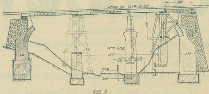
MOST TYMCZASOWY DLA 1. FAZY ODBUDOWY. PRZEKRÓJ PODŁUŻNY
