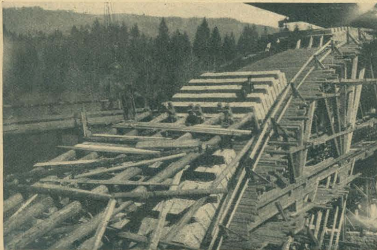
Rys. 12. Widok w czasie układania ciosów I pierścienia.
