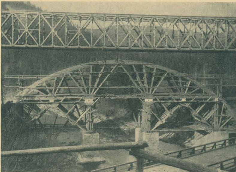
Rys. 10. Widok rusztowań krążynowych.
