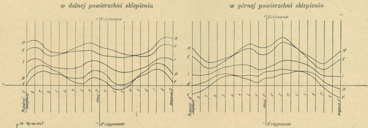
Wykres natężeń w nowym sklepieniu.
