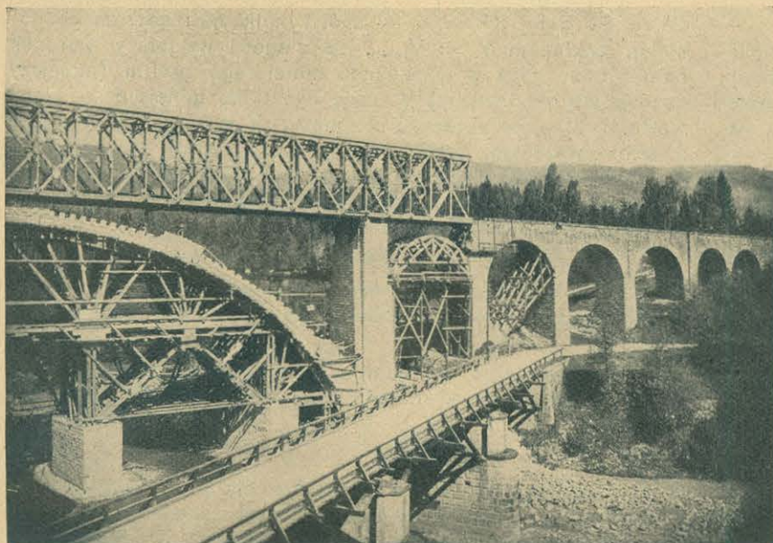
Rys. 13. Widok sklepienia w czasie układania III pierścienia.
