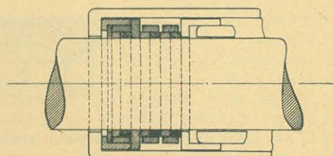
Pierwotny układ szczeliwa syst. Jasińskiego
