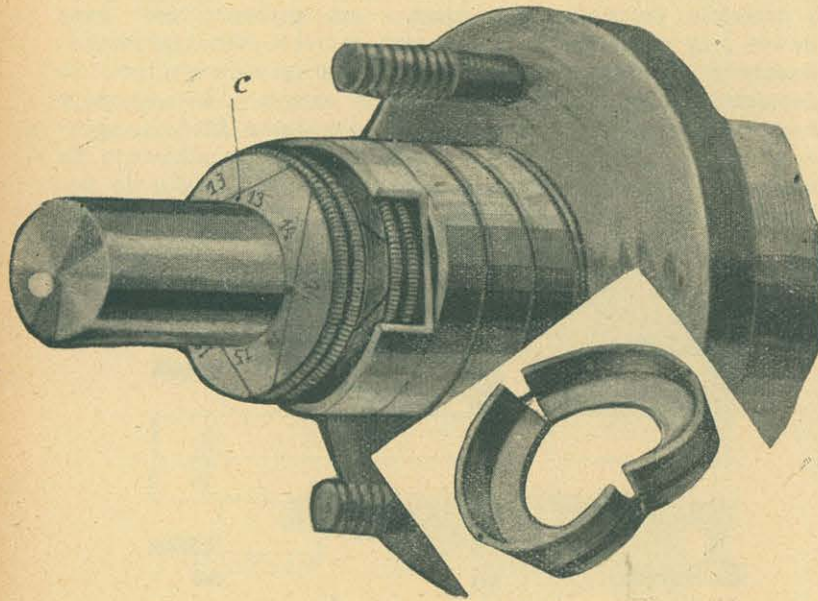
Rys. 7 Szczeliwo „Pacyfic“.
