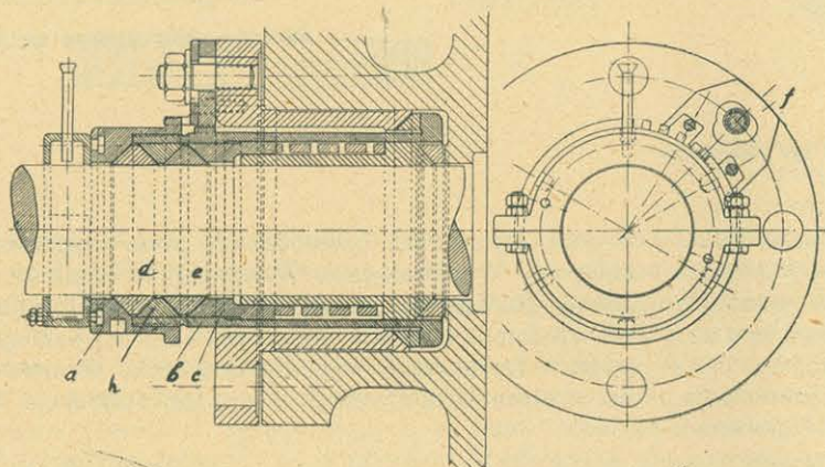
Rys. 2. Dławnica systemu Henke.
