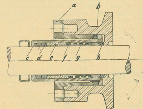
Rys. 1. Dławnica systemu Schmidta.
