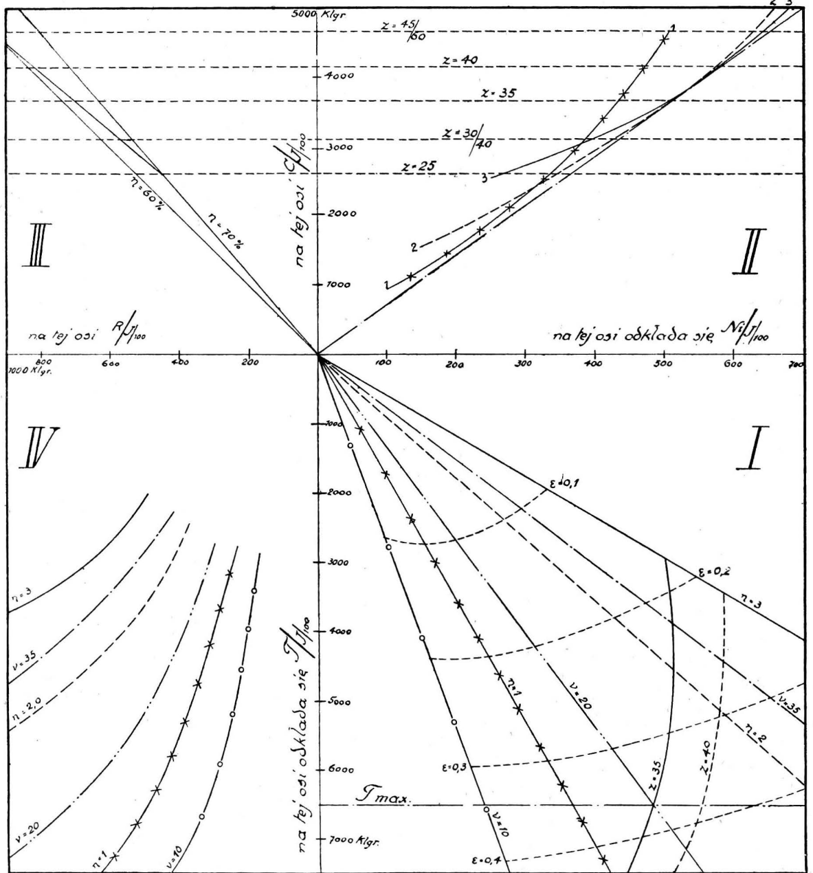
Tablica pracy parowozu i rozchodu węgla.
