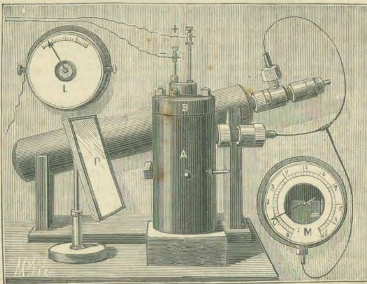
Fig. 1. Przyrząd Cailleteta. A Bryła stalowa z wydrążeniem walcowym. — P zwierciadło. — M manometr. — L amperometr.
