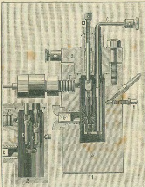
Fig. 2. Przecięcie przyrządu Cailleteta. 1) Urządzenie do utrzymania łuku elektrycznego. Węgiel odosobniony E wydrążony jest w postać tygielka. 2) Urządzenie z drutem platynowym skręconym spiralnie.
