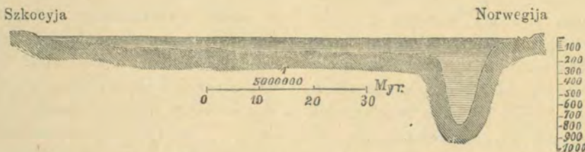
Fig. 4. Profil dna morza Północnego, od północnego krańca Szkocji do Stavanger w Norwegii. Skala długości ( 1/5,000,000 ) 200 razy większa, aniżeli skala wysokości.
